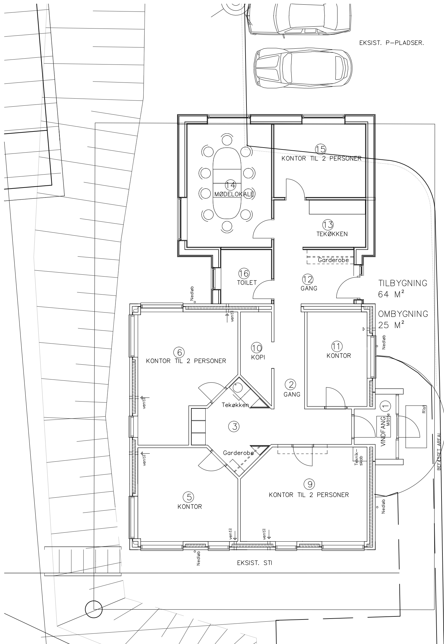
STUEPLAN MÅL 1:100
