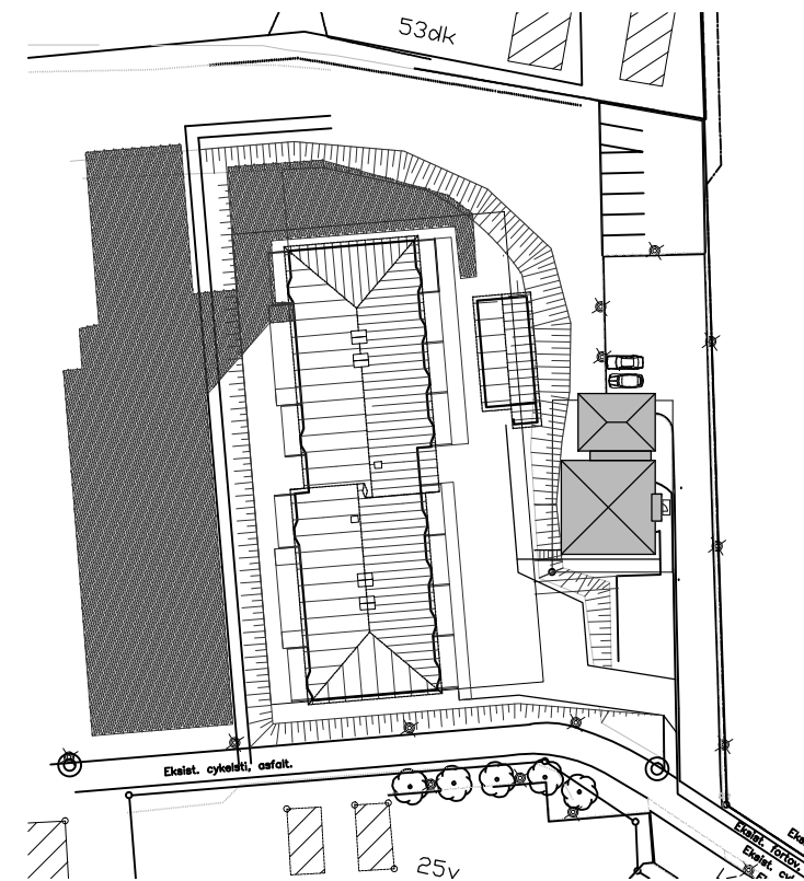
SITUATIONSPLAN MÅL 1:1000
